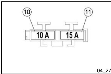
Sicherungshalter «C».
